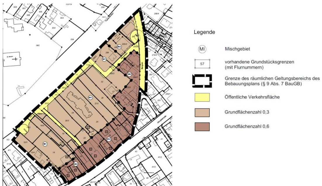
Abb: Aufteilung des Baugebiets nach dem Maß der baulichen Nutzung
